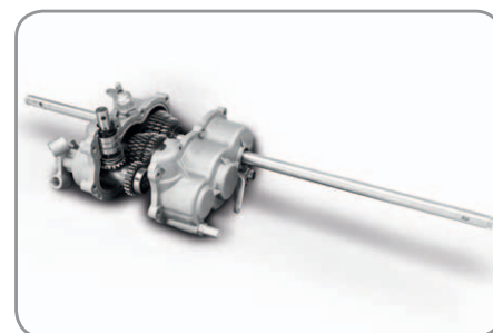
3-Gang-Getriebe mit Kardanwelle
