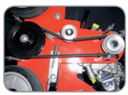
Langlebiger Messerwellenantrieb mit kugelgelagerter Metallspannrolle. Doppelriemen
