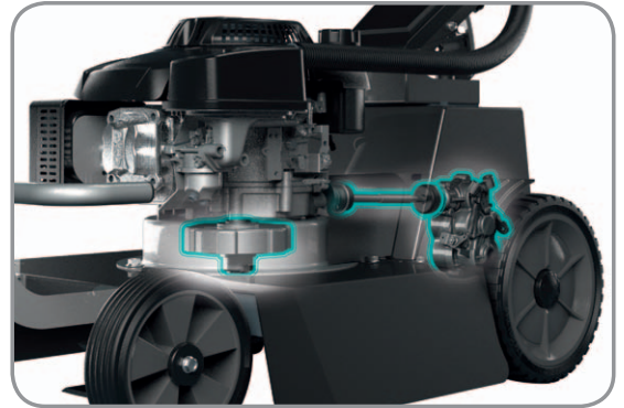
Kurbelwellenschutz / Kardanwelle
