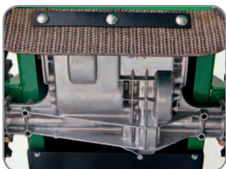
Robustes Getriebe mit integriertem Differenzial bei dem BC 2601 HHC EU
