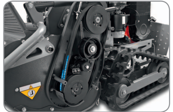
Doppelriemen für perfekten Kraftschluss
