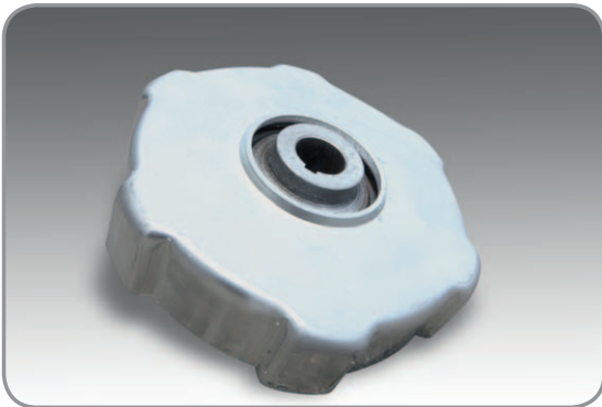
Sicherheitsgummipuffer mit Aluminiumverschalung zum Schutz der Kurbelwelle
