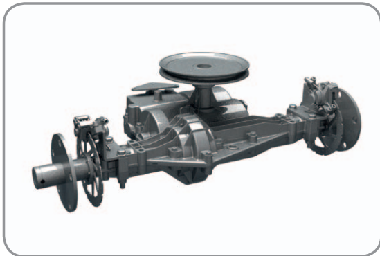
Vollprofilgetriebe mit integriertem Radbremssystem
