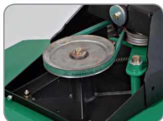
Überdimensionierter und wartungsfreier Messerantrieb
