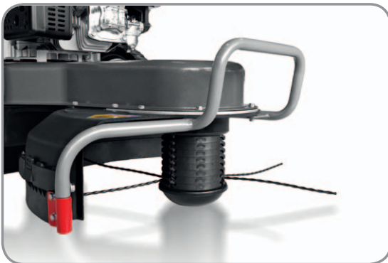
Die Trimmerspule ist auf einer Kernwelle gelagert. Somit kein nennenswerter Verschleiß
