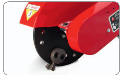
Enorm hartes Fräswerk mit einzeln austauschbaren Fräszähnen.
