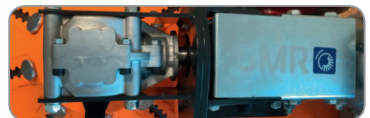
Kardanwelle mit Alu-Winkelgetriebe.
