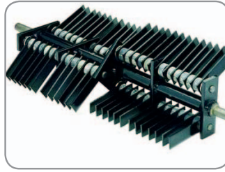
Vertikutierwellen mit Pendelmessern als Serienausstattung.
