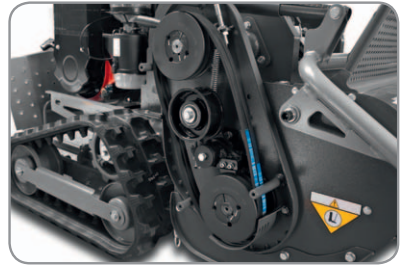
Doppelriemen für perfekten Kraftschluss
