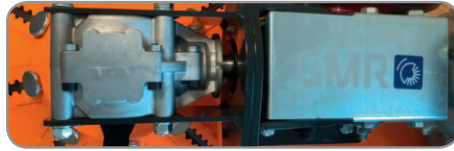
Kardanwelle mit Alu-Winkelgetriebe.
