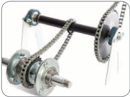
1,25" Kegelachse mit wasserdichten 2" Kugellagern im Zusammenspiel mit einer gepanzerten Antriebskette.
