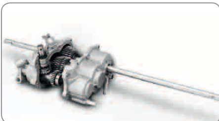
Dreigang-Schaltgetriebe mit direkter Kardananbindung und enorm hoher Standzeit.
