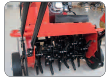
30 gehärtete Hohlzinken mit 7 cm Arbeitstiefe.
