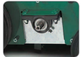
Abschmierbare, robuste Wellenlager.
