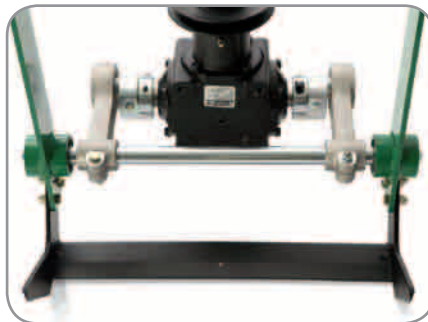
Gusseisernes Spiralgetriebe, wasserdichte Lager, 1" große Seitenstabilitätsstange in Verbindung mit überdimensionierter Aluminiumaufhängung in Exzenteranordnung für herausragende Festigkeit. Laserplattiertes Messer für präzise Schnitte und die dreifache Lebensdauer.
