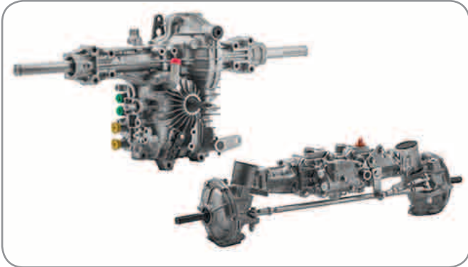
Tuff Torq™ 4WD Hydrostaten. Verteilen die Kraft dort hin, wo sie benötigt wird.
