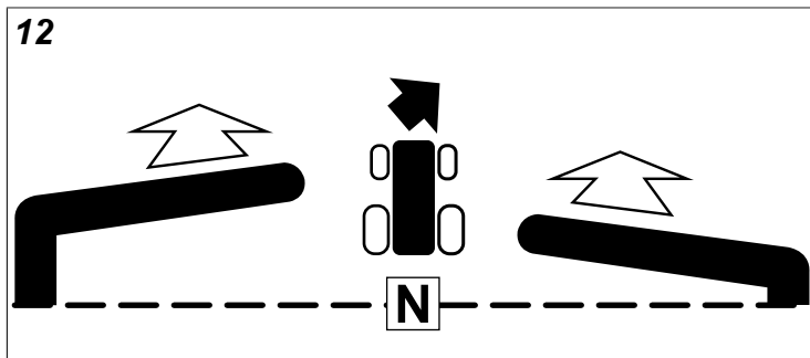
Für eine sanfte Rechtsbewegung den linken Fahrsteuerungshebel weiter nach vorne schieben als den rechten Fahrsteuerungshebel.
