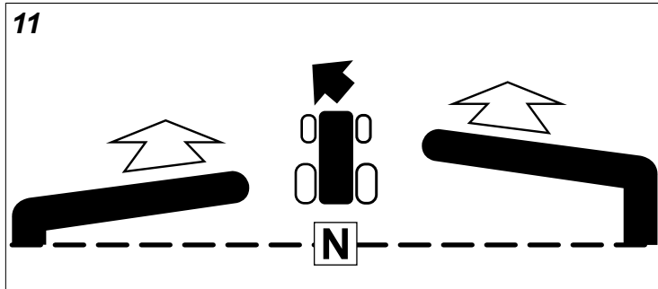
Für eine sanfte Linksbewegung den rechten Fahrsteuerungshebel weiter nach vorne schieben als den linken Fahrsteuerungshebel.
