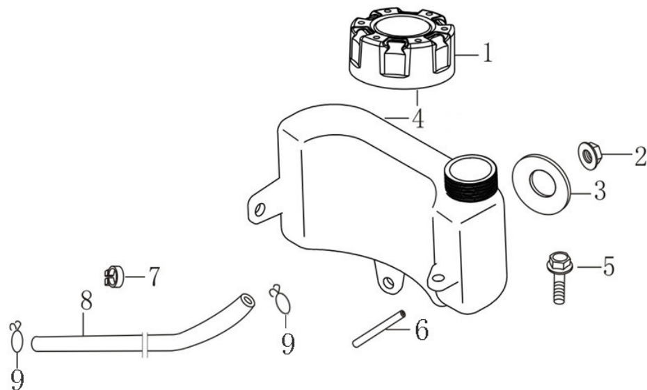
燃油箱 (FUEL TANK)
