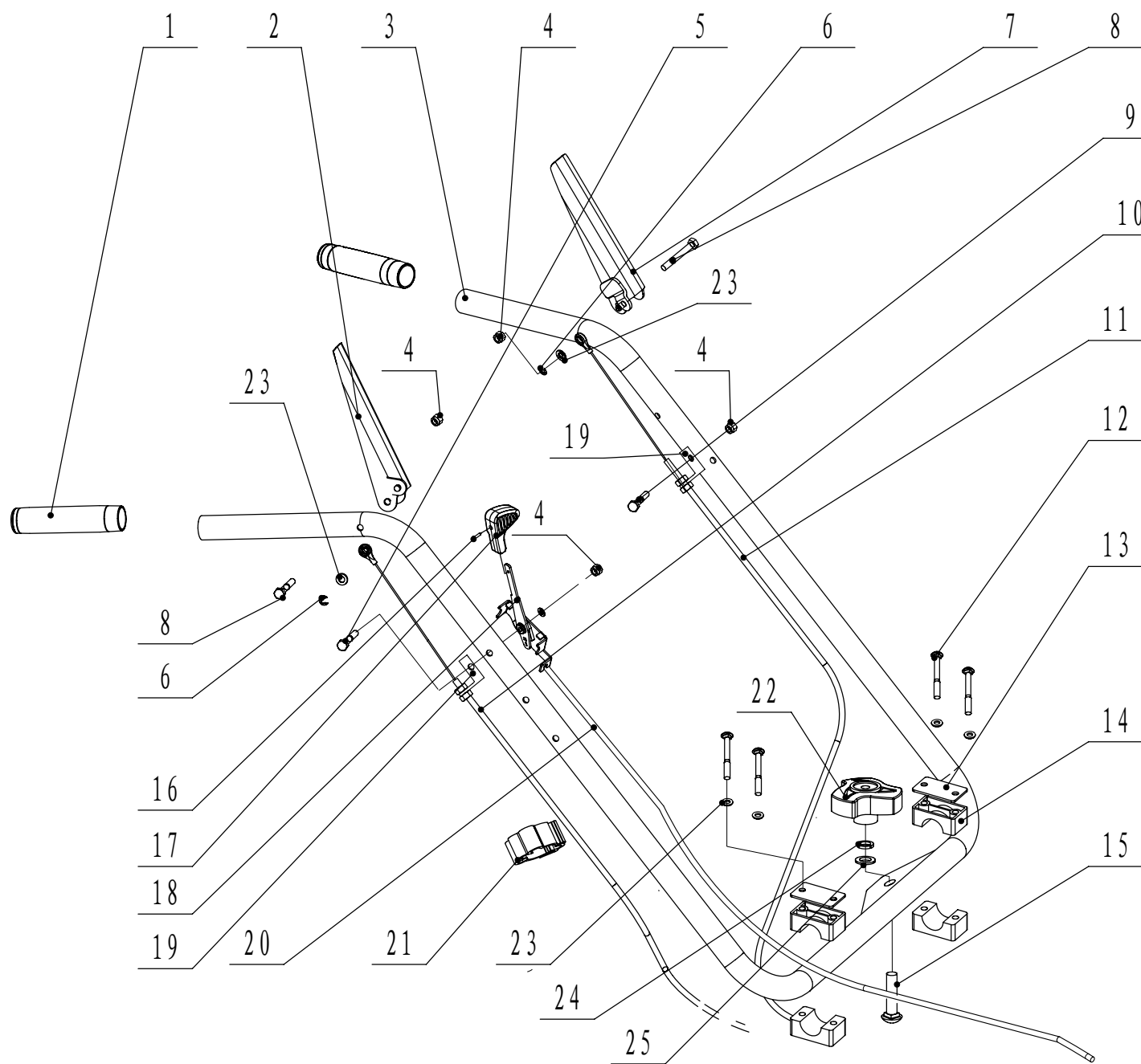
BSW806B0100000把手部分爆炸图
