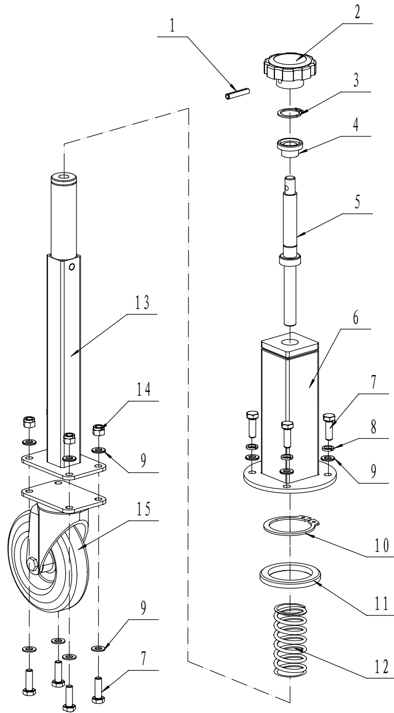
BSW705C0200000升降器部分爆炸图
