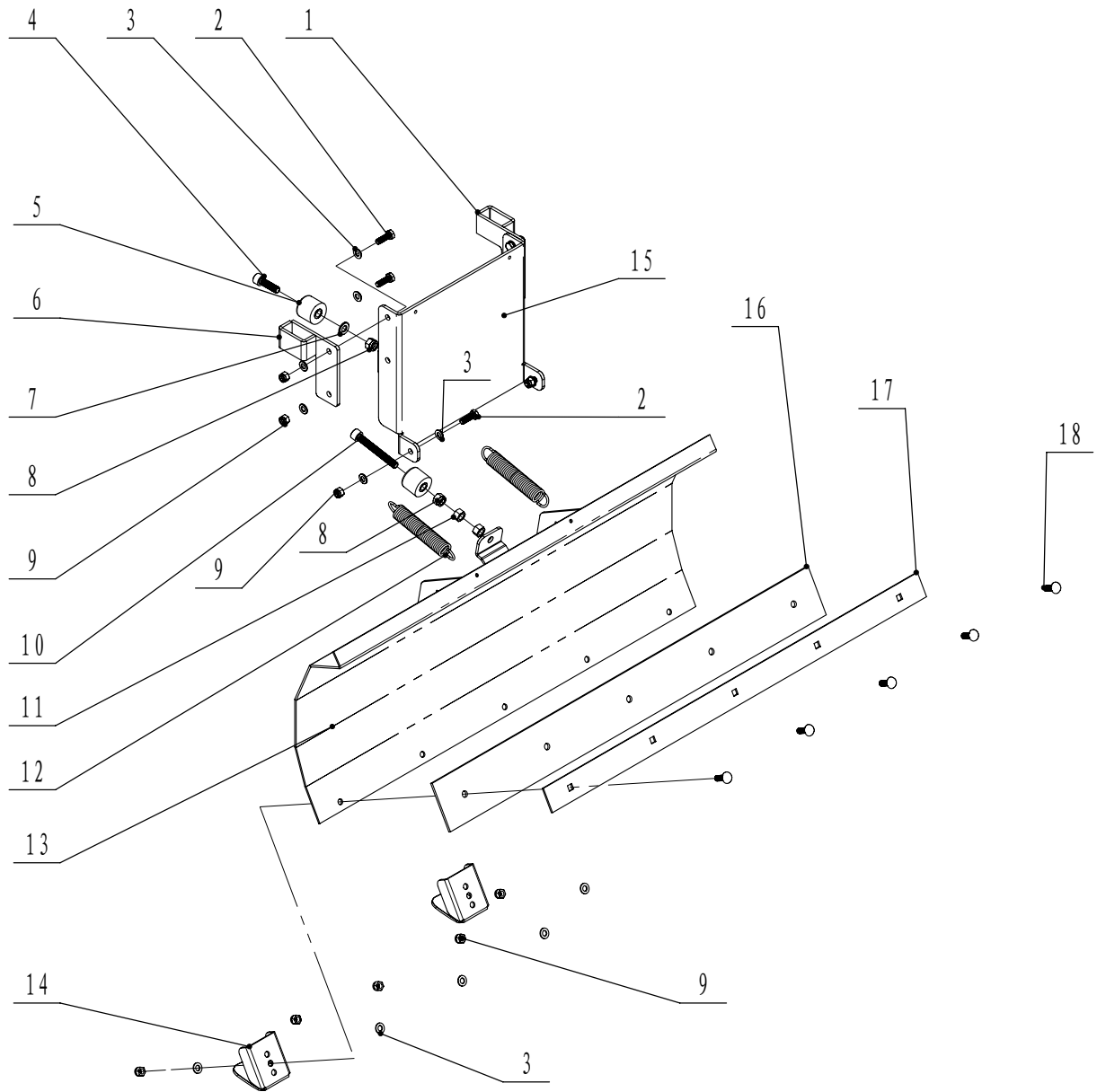
BSW806B0900000推雪装置爆炸图
