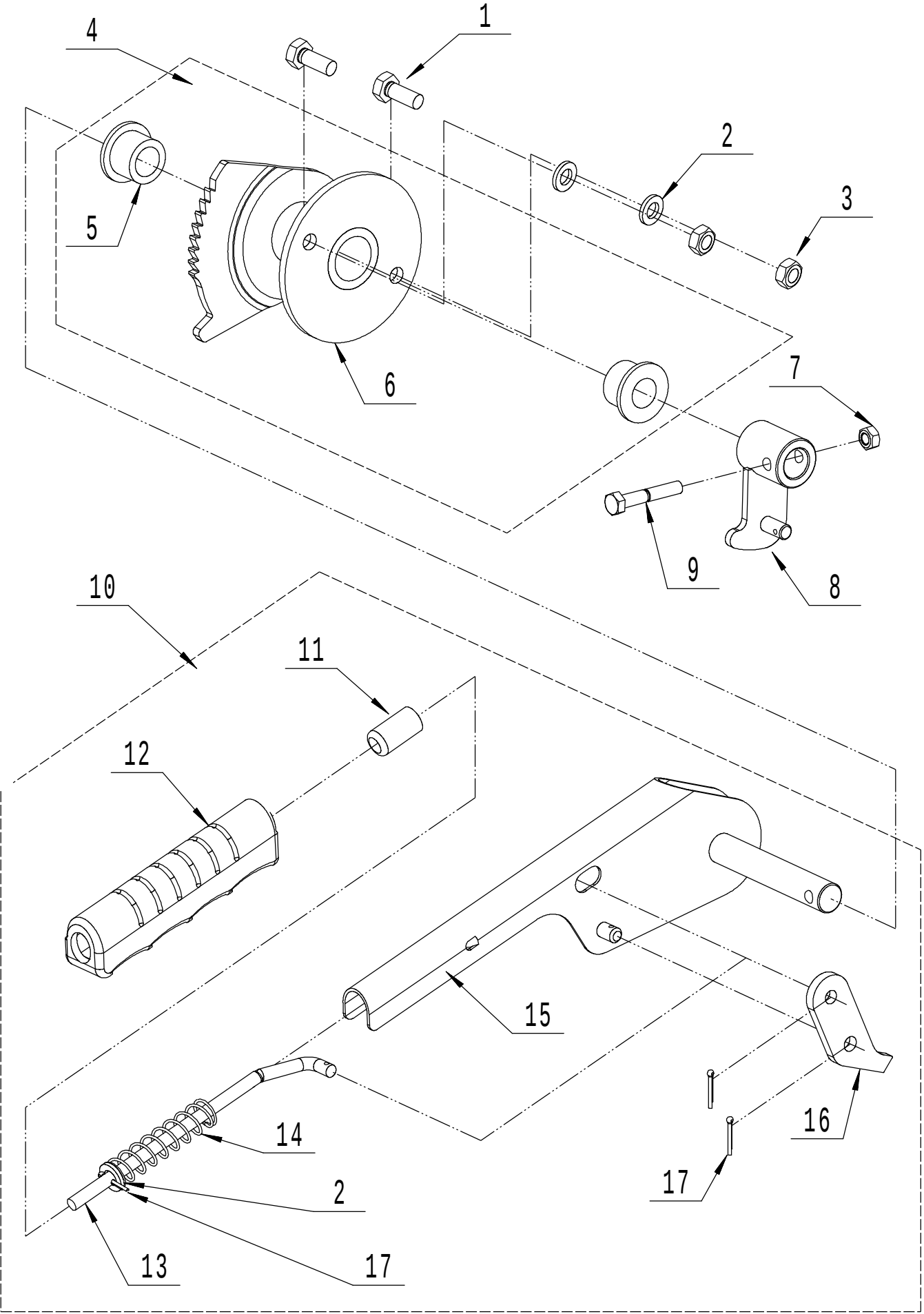
5: 驻车机构
